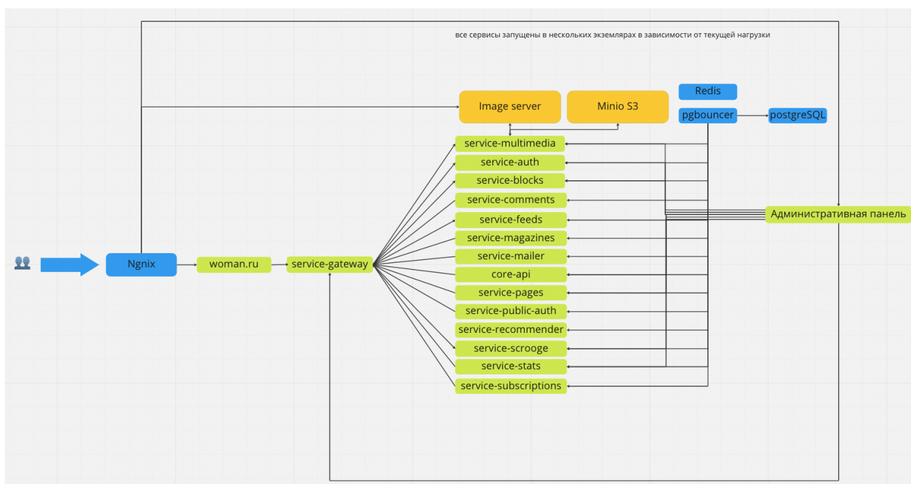
Рис. 1. Общая схема ПО
